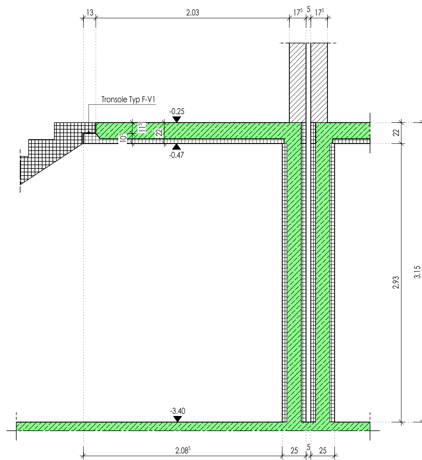
Schnitt 3-3 M 1:25
