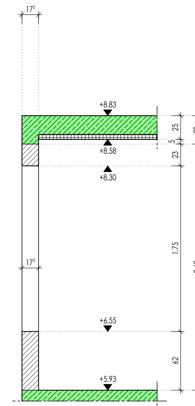
M 1:25
