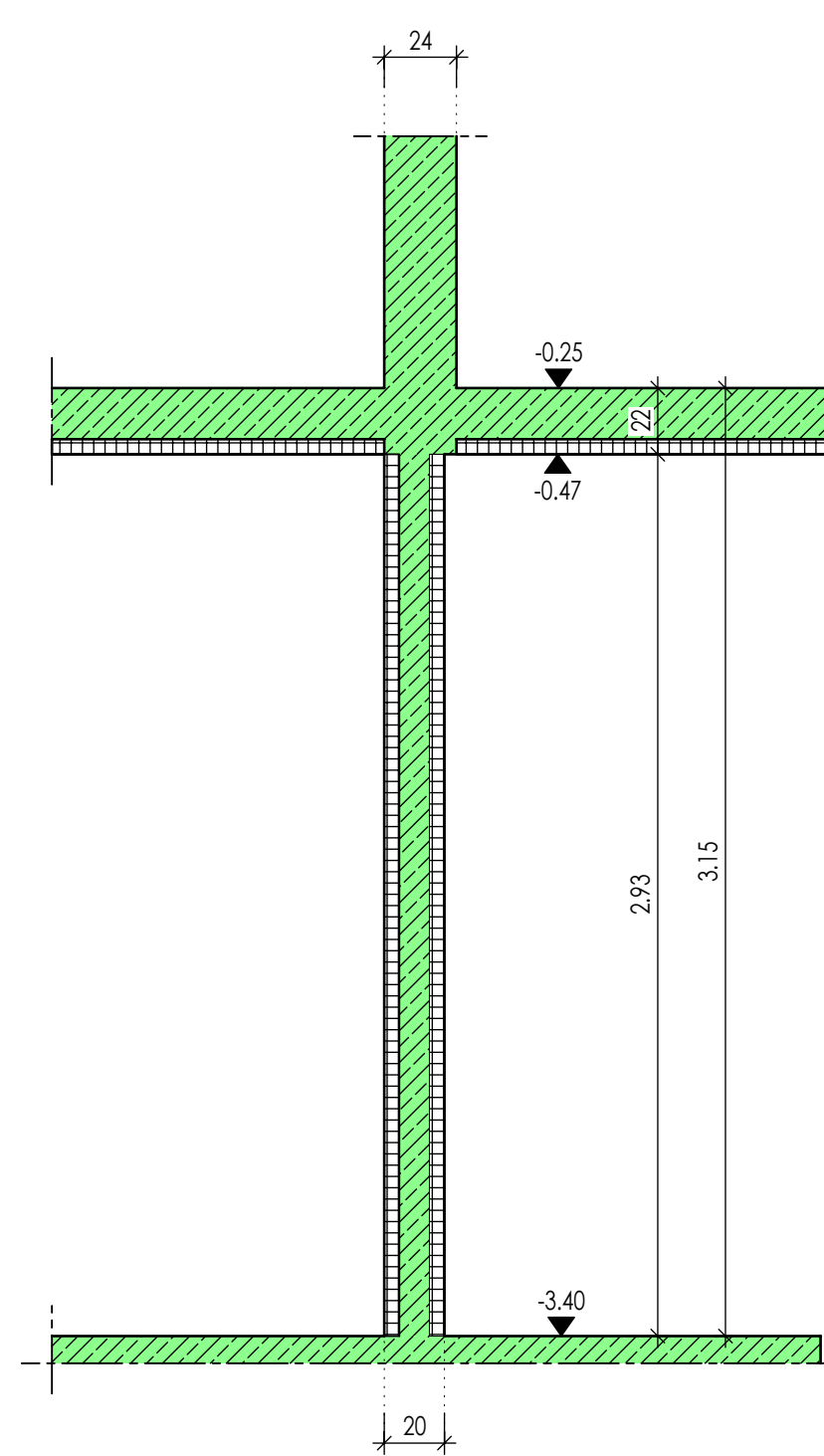
Schnitt 2-2 M 1:25
