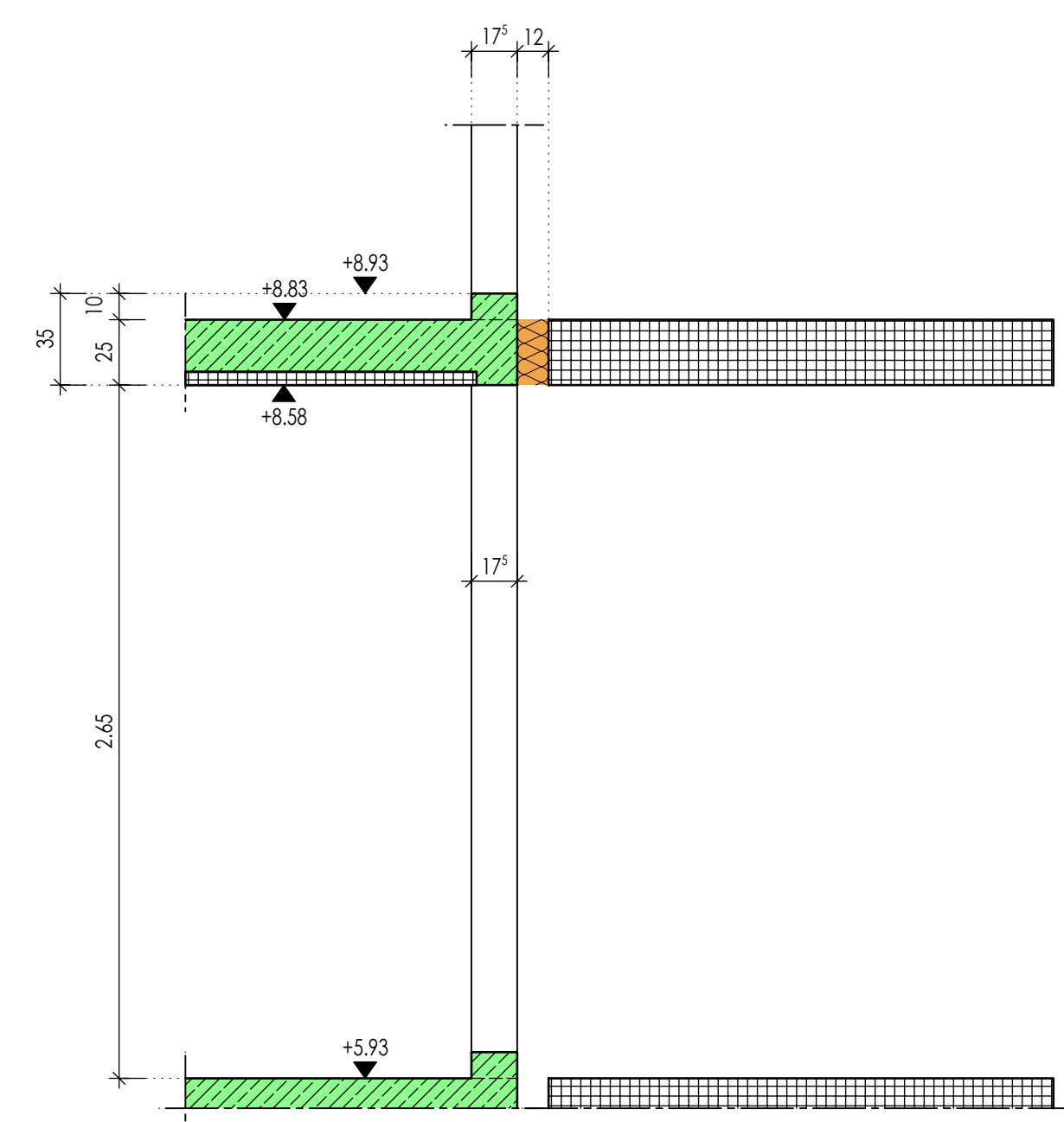
M 1:25
