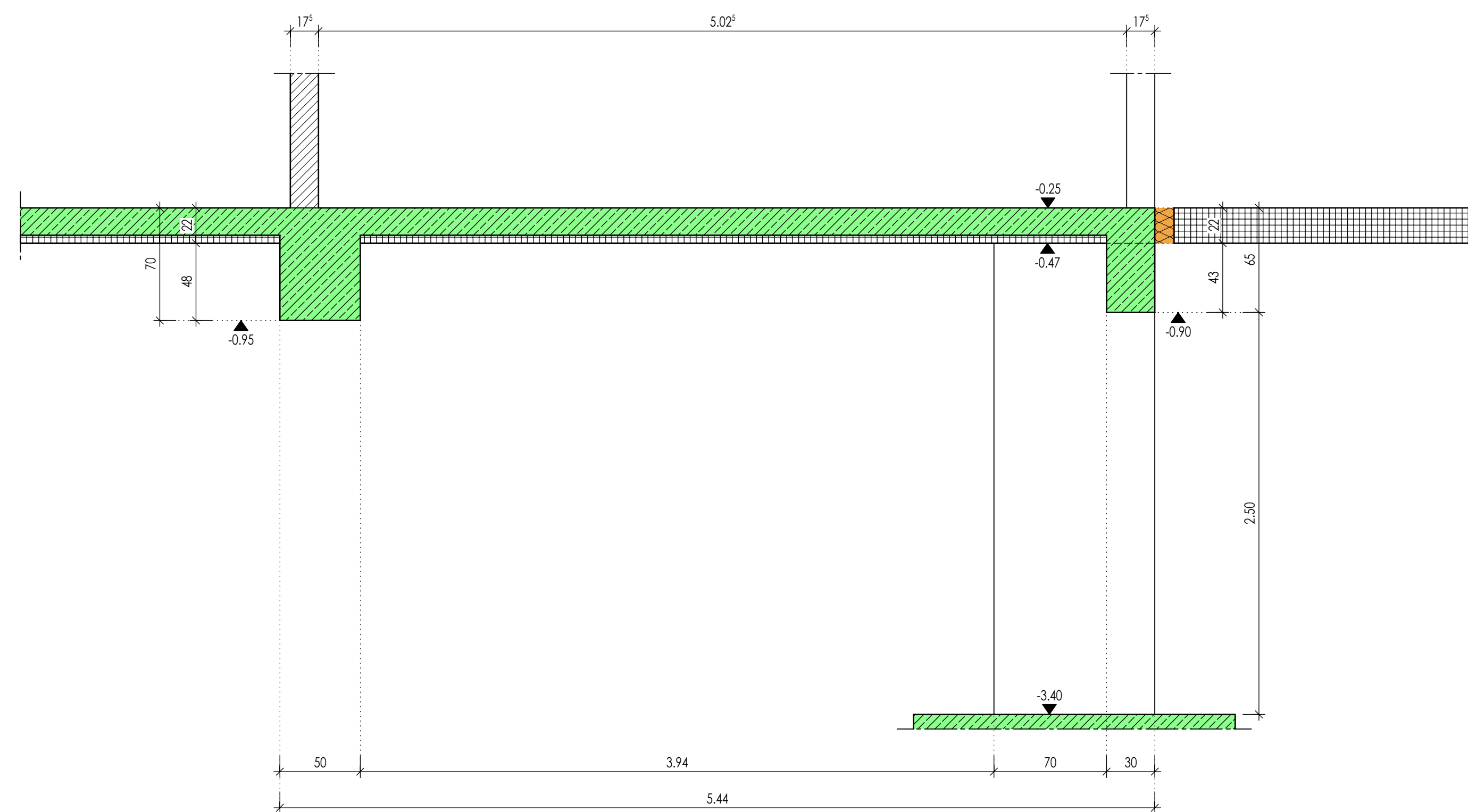
Schnitt 3-3 M 1:25
