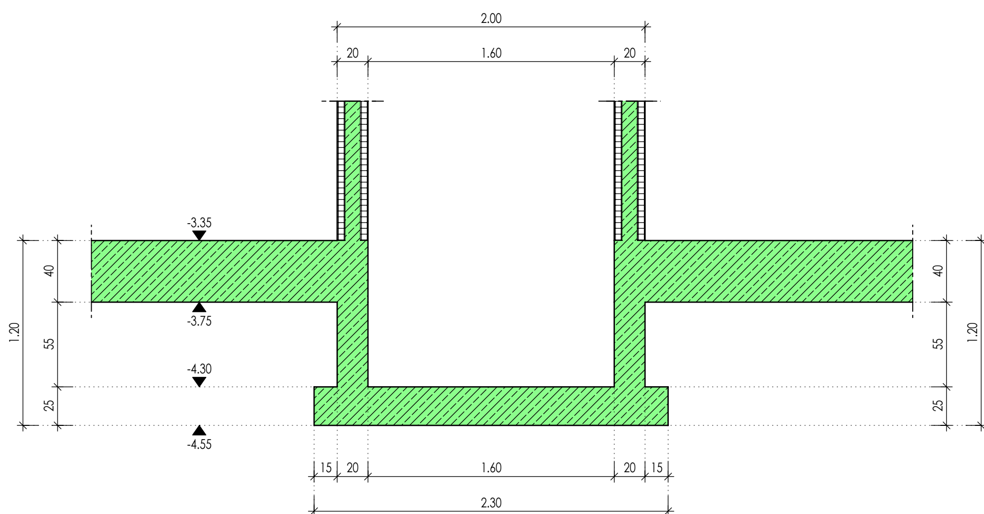
M 1:25
