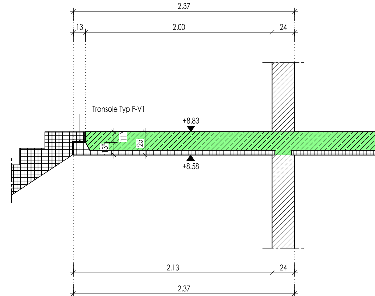
M 1:25
