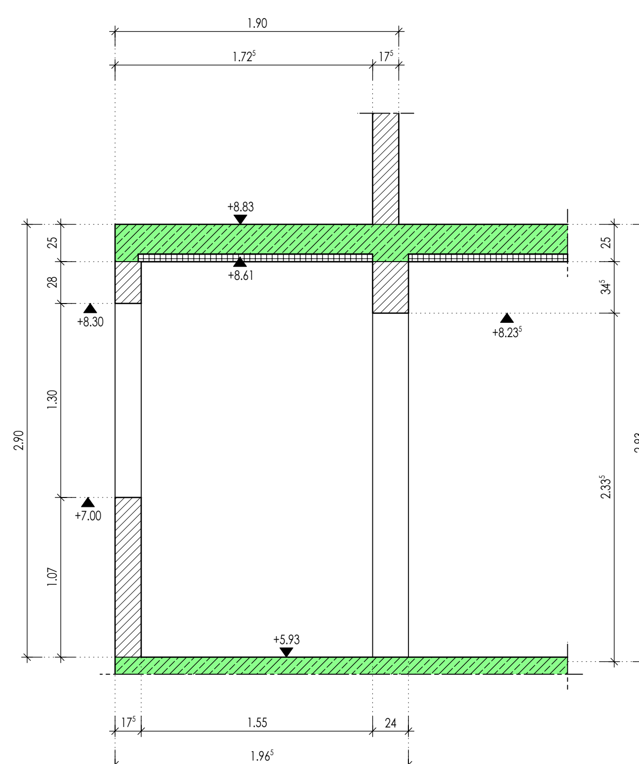
M 1:25
