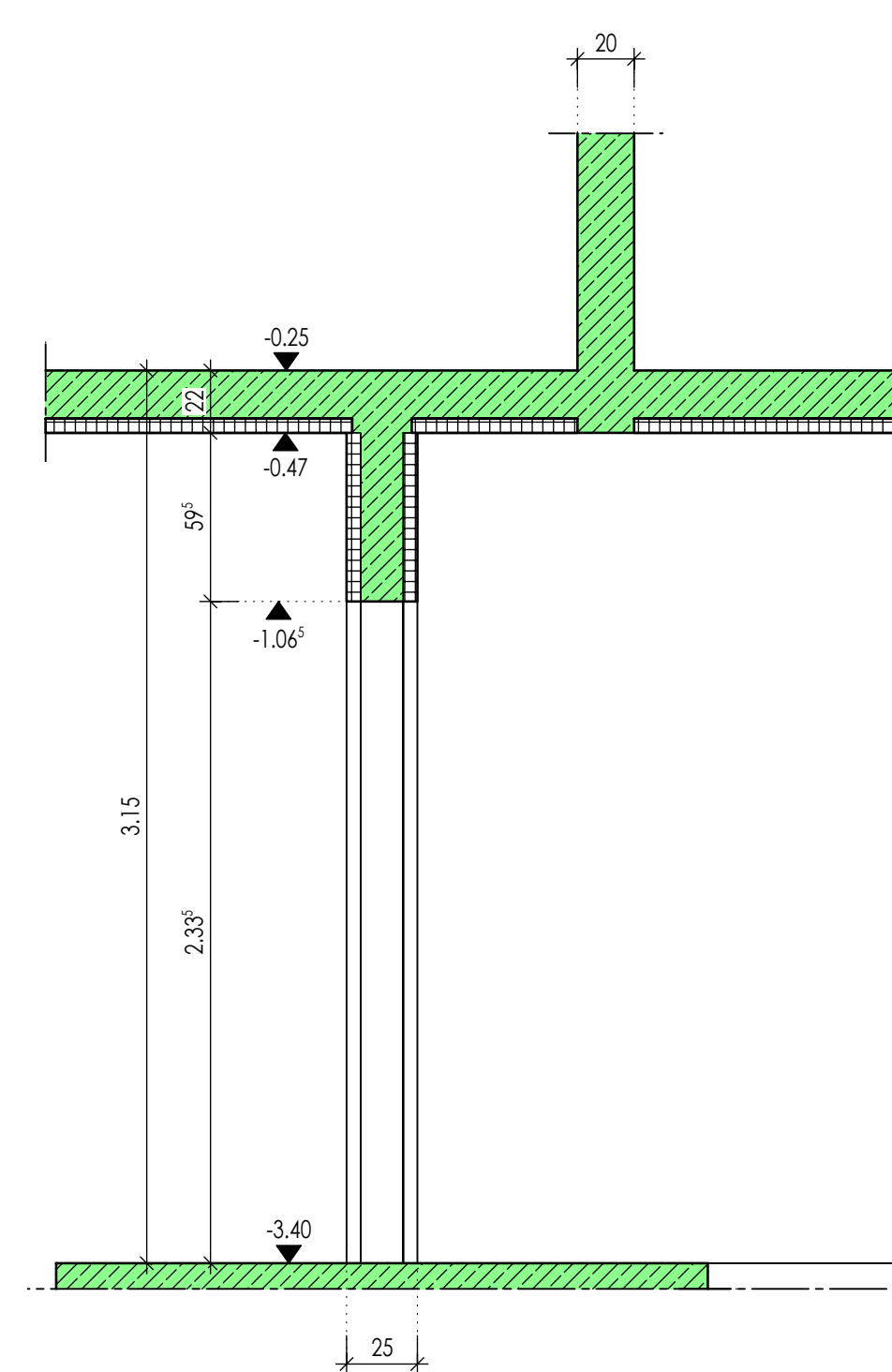
Schnitt 4-4 M 1:25
