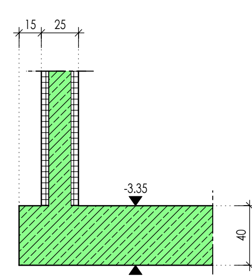
M 1:25
